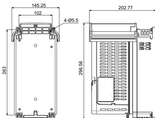
ATV610D18N4A, ATV610D22N4A
