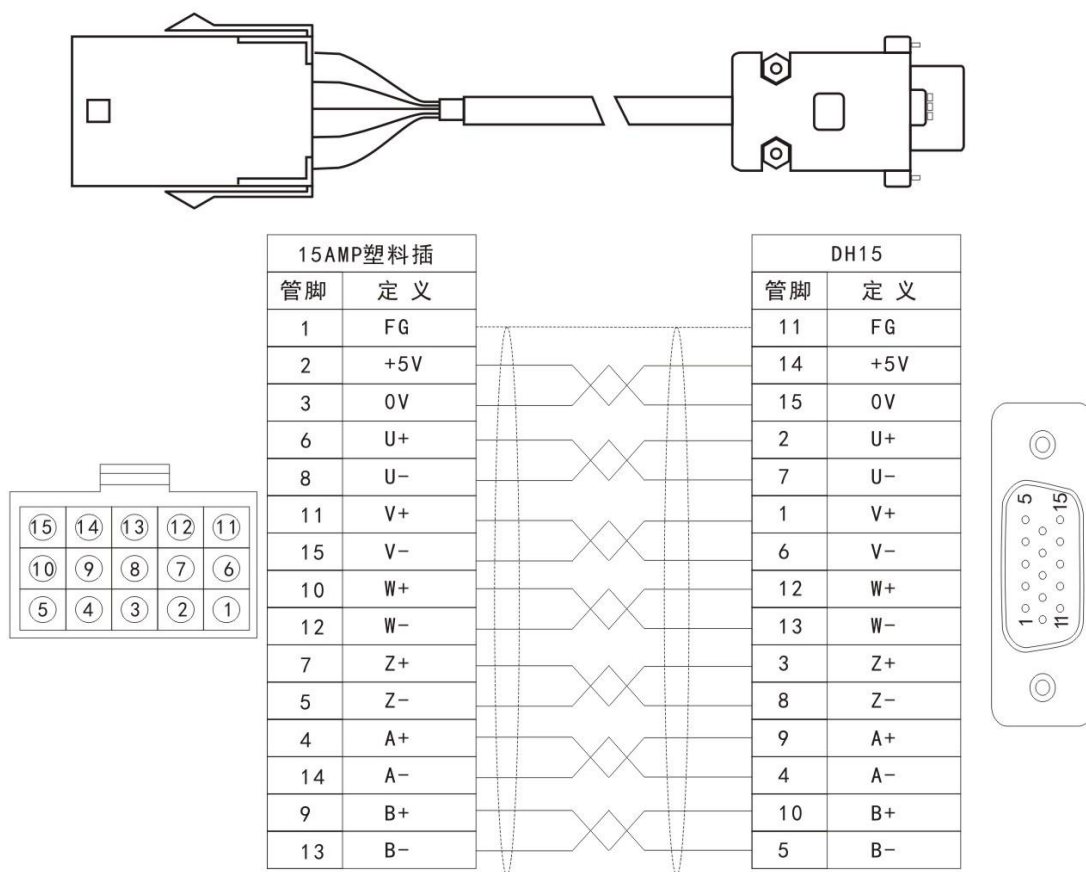
图 2.3 14 线编码器电缆接线示意图
