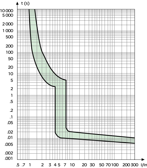
C65H-DC B 曲线
