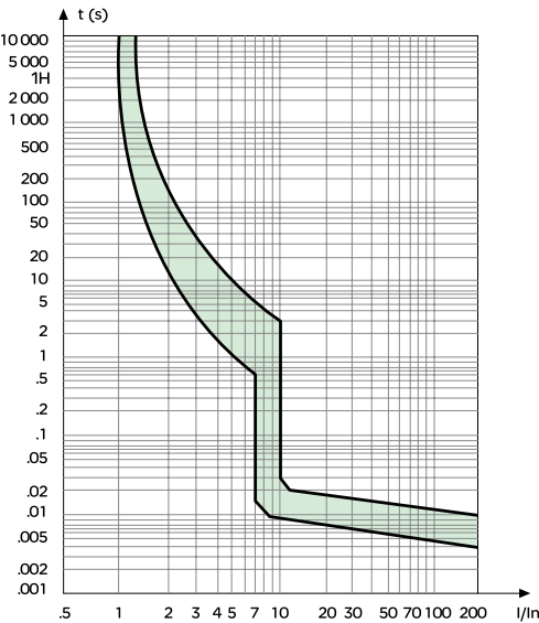
C65N-DC/C65H-DC/C65L-DC C 曲线
