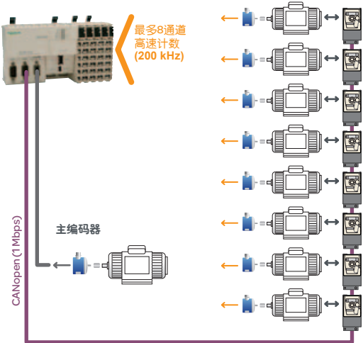
高速计数器功能(单相或双相)
