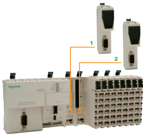
1 TM5 PCRS●通讯模块：Modbus/ASCII串行链路 2 TM5 PCDPS通讯模块：Profibus DP从站链路 用于安装到M258逻辑控制器或LMC058运动控制器中两个闲置PCI插槽上
