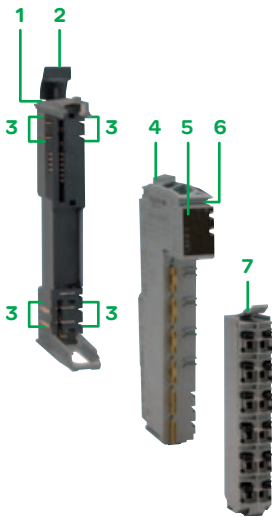
接收器单片式远程I/O模块
