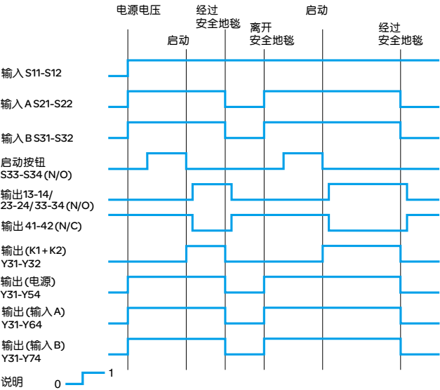
带有监控启动的安全地毯和边沿开关监控功能
