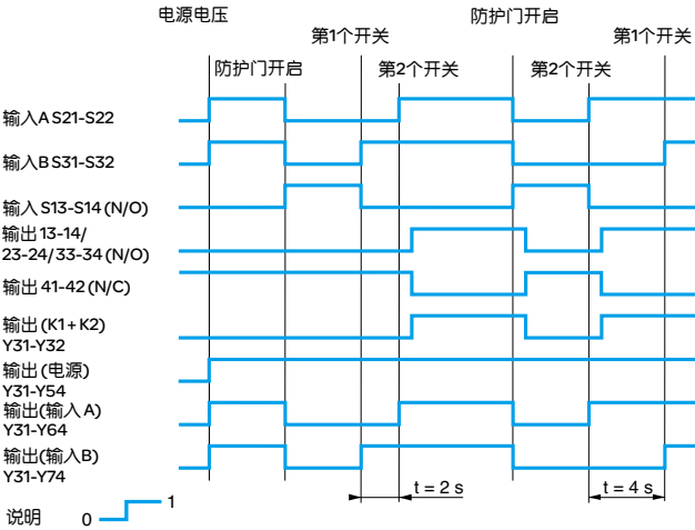
带有固态输出的光幕监控功能 (ESPE)
