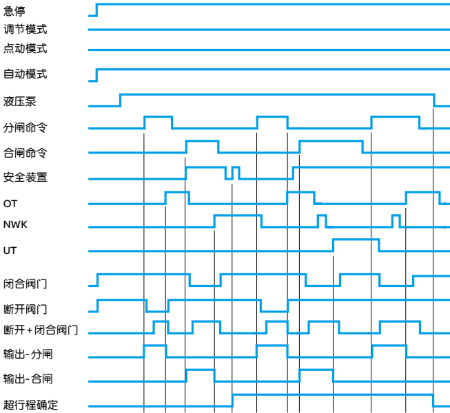
液压机，模式=自动，带超行程监控以及自动化平台的分闸和合闸控制
