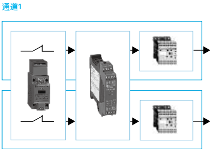
符合EN/ISO 13849-1标准的功能框图
