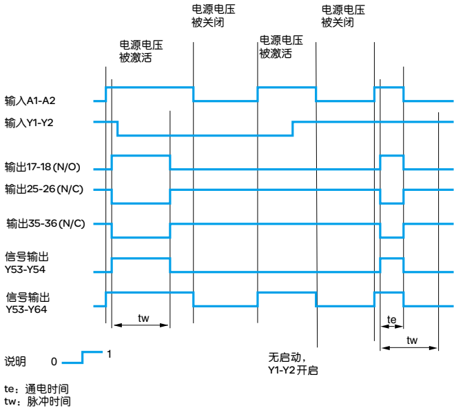
XPSTSW模块的逻辑图
