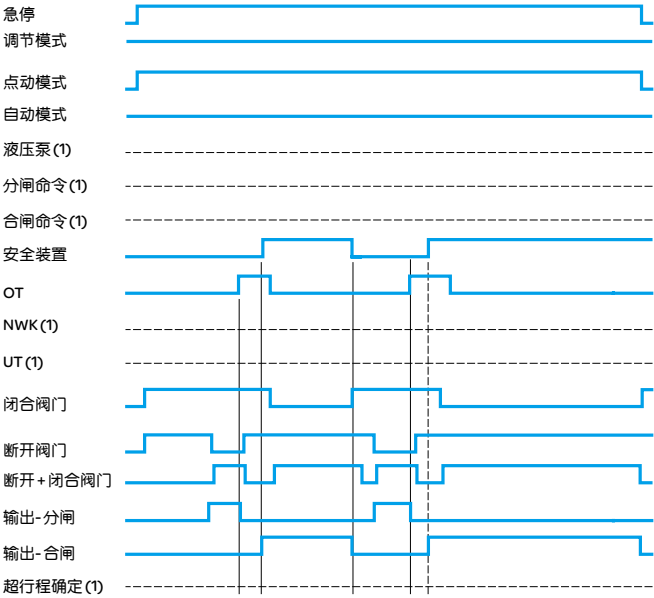
液压机，模式=点动
