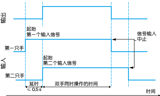
双手操作台的功能图
