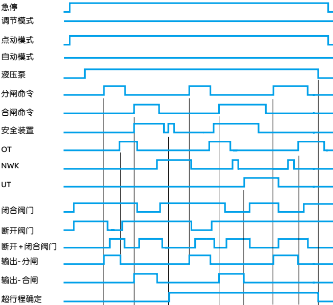
液压机，模式=点动，带超行程监控以及自动化平台的分闸和合闸控制
