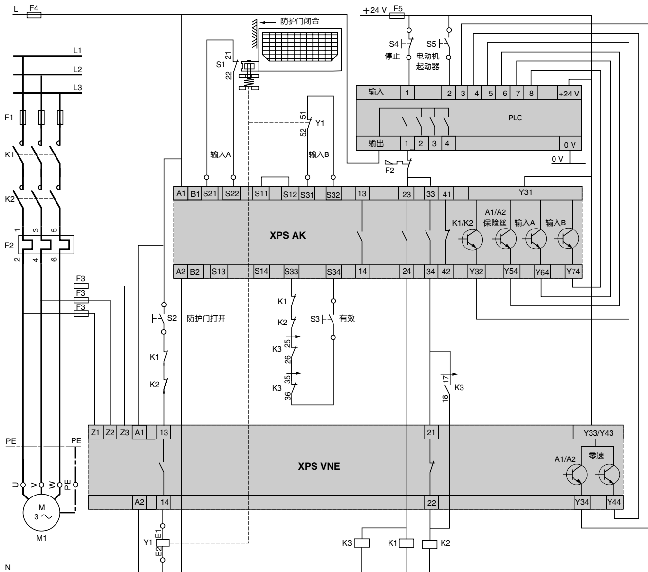
S1+Y1: 去电时有电磁锁定功能的防护门开关, XCS E型或XCS L型 去电时的脉冲XPS TSW继电器
