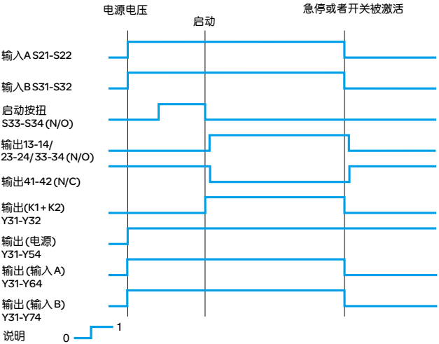
带有监控启动的安全地毯和边沿开关监控功能
