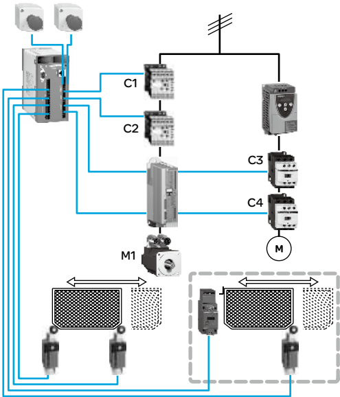
印刷机械中与安全有关的部分(计算是根据灰框中的电路得出)
