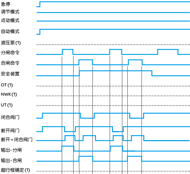
液压机，模式=自动
