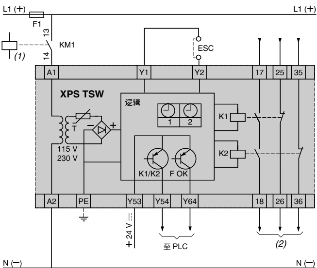
接线图
