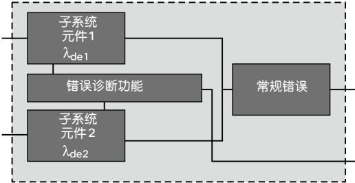
D类子系统的结构
