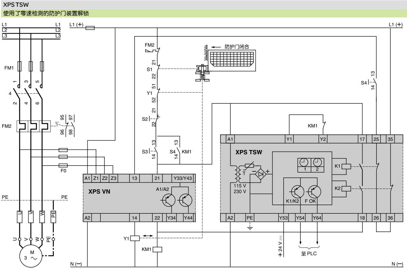
接线图
