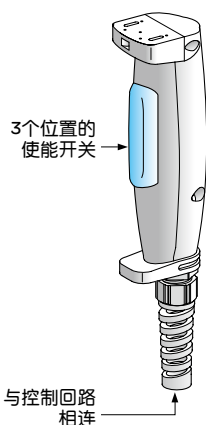
使能开关XY2AU1: 2个使能功能, 3个位置+1N/C
