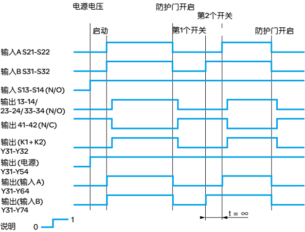
急停监控或者开关监控功能
