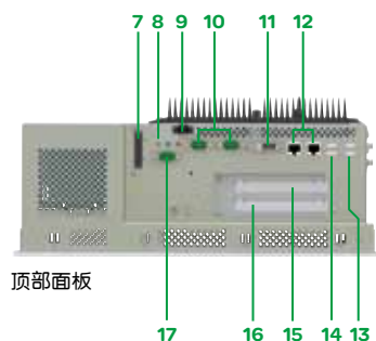
Magelis平板电脑, 15"或19", 2个PCI插槽
