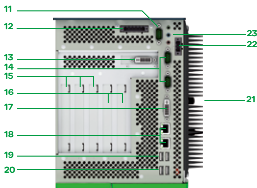
Magelis箱式工控机的顶部面板 5个PCI插槽
