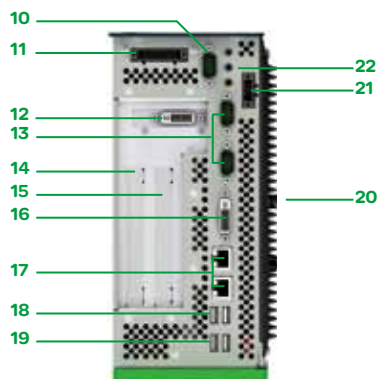
Magelis箱式工控机的顶部面板，2个PCI插槽
