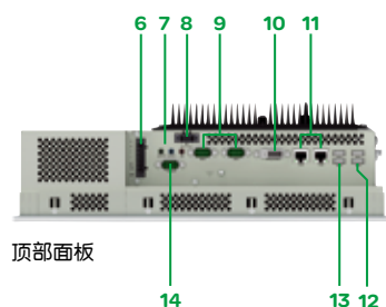
Magelis平板电脑, 15"或19", 无PCI插槽
