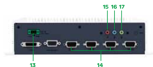
UNIVERSAL MAGELIS小型箱式工控机后视图
