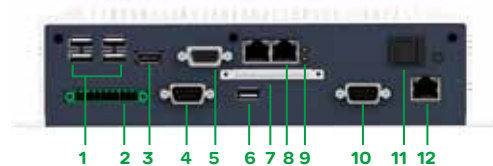
UNIVERSAL MAGELIS小型箱式工控机前视图
