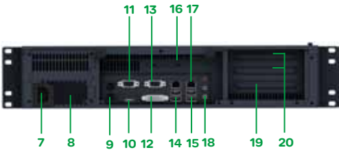
Universal Magelis机架式电脑后视图
