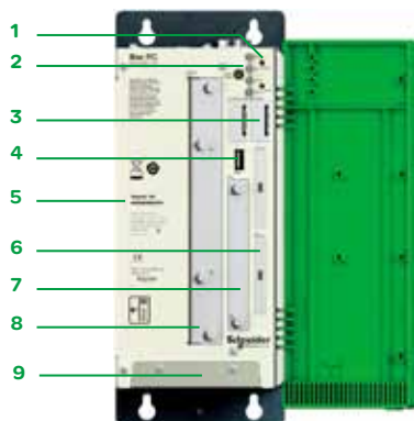
Magelis箱式工控机的前面板，门打开 2个PCI插槽
