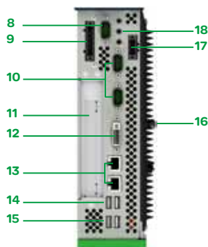
Magelis箱式工控机的顶部面板，1个PCI插槽
