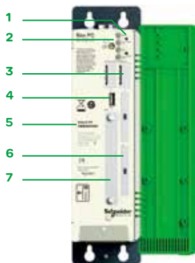
Magelis箱式工控机的前面板，门打开 1个PCI插槽
