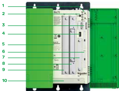
Magelis箱式工控机的前面板，门打开 5个PCI插槽
