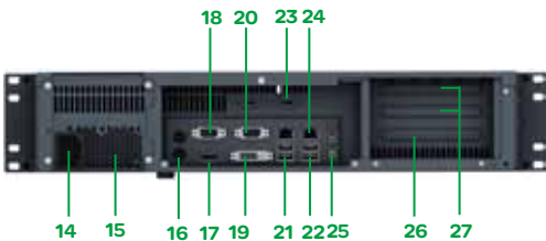
Optimized Magelis机架式电脑后视图
