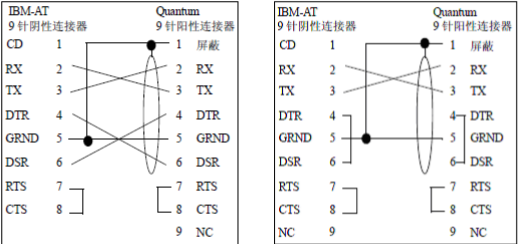
台式计算机Modbus端口引脚连接 便携式计算机的 Modbus 端口引脚连接
