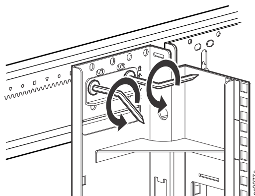
750 mm 宽机柜
