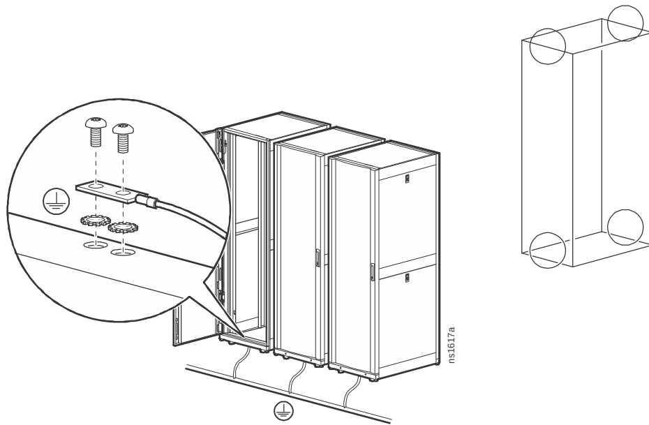
机柜上的接地位置
