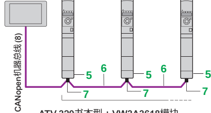
ATV 320书本型 + VW3A3618模块
