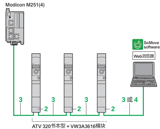
ATV 320书本型 + VW3A3616模块
