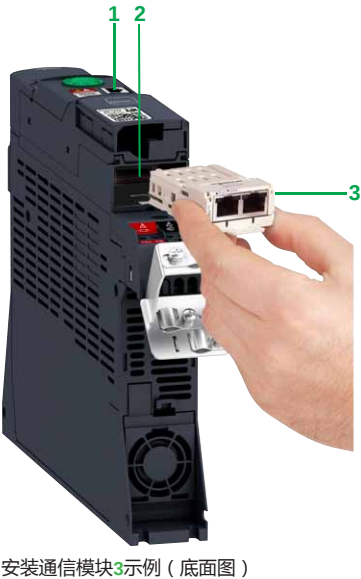
安装通信模块3示例（底面图）
