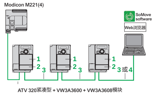
ATV 320紧凑型 + VW3A3600 + VW3A3608模块
