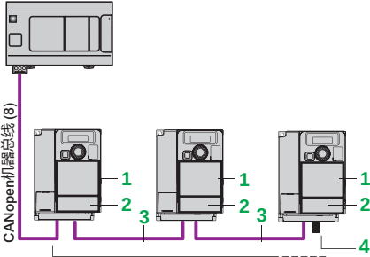
ATV 320紧凑型 + VW3A3600 + VW3A3608模块
