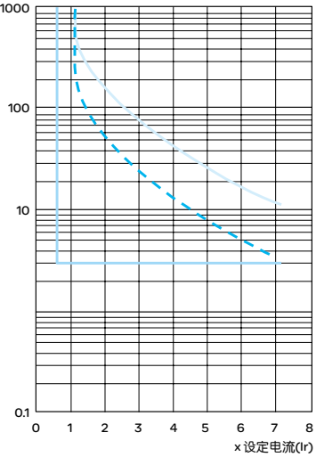
类别 20 的脱扣曲线
