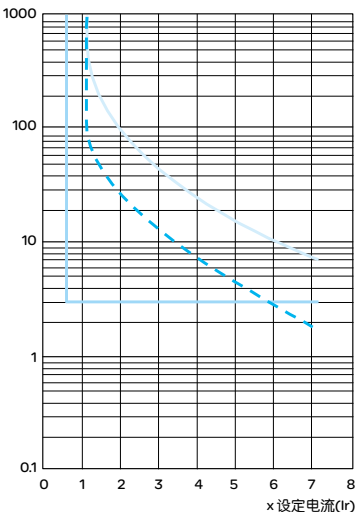
类别 30 的脱扣曲线
