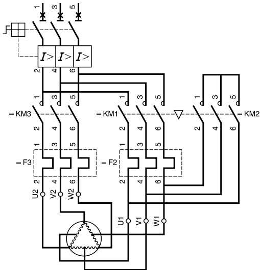
变极 GV2LE
