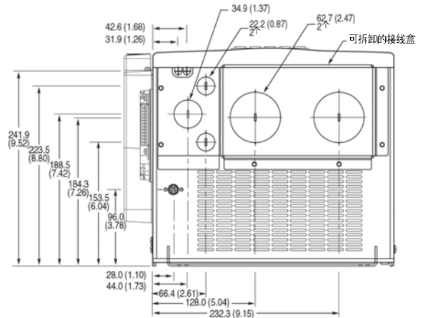
5型框架 - 100 HP, 480V(55 kW, 400V)标称负载变频器
