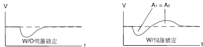
阶跃负载速度响应
