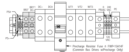
5型框架—100HP标称负载 650V 直流输入
