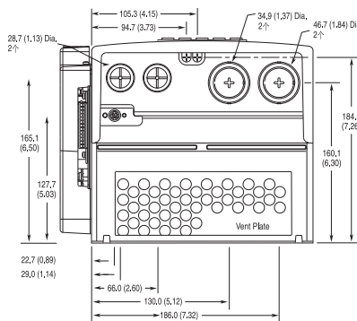
3型框架 - 50 HP, 480V(37 kW, 400V) 标称负载变频器
