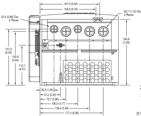
2型框架(底部视图)
