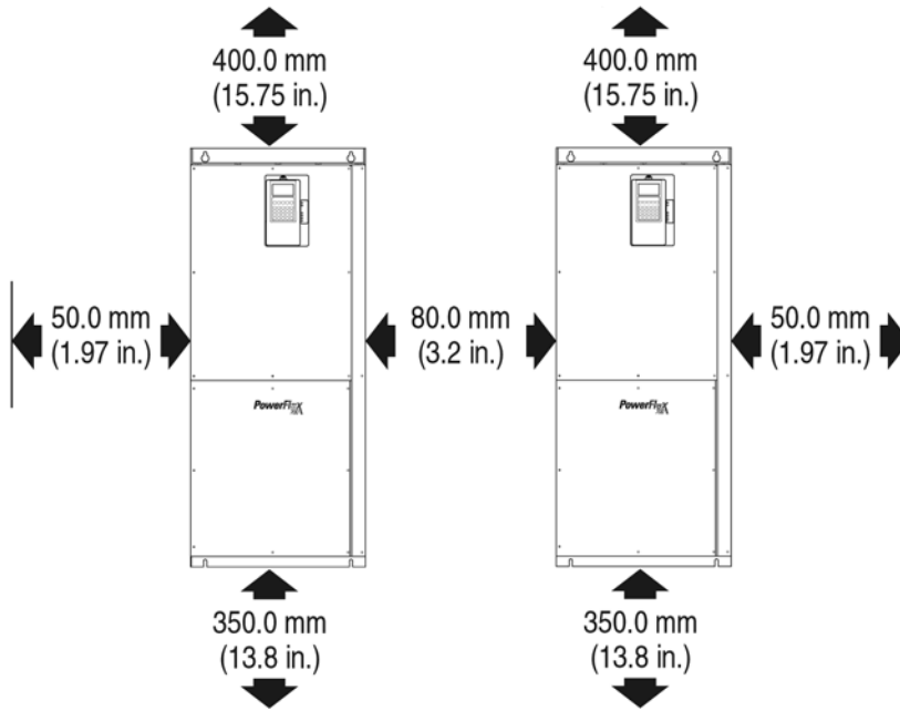
9 型框架
