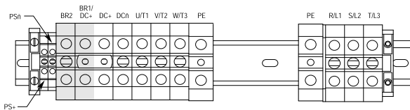
5型框架—75HP标称负载 480V 交流输入
