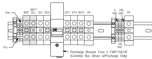
5型框架—75HP标称负载 650V 直流输入
