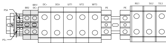
5型框架—100HP标称负载 480V 交流输入
