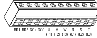
3和4型框架
