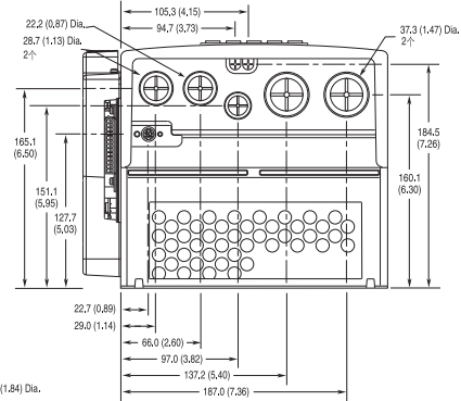
3型框架 - 除50 HP, 480V(37 kW, 400V)之外的所有变频器。
