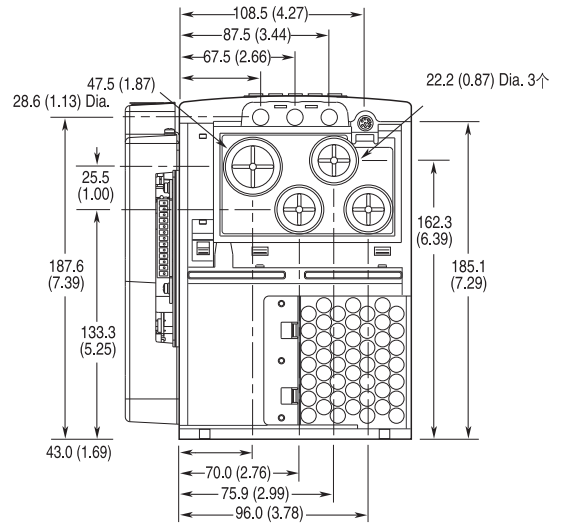
3型框架 - 除50 HP, 480V(37 kW, 400V)之外的所有变频器。
