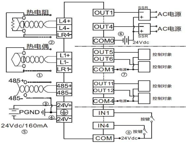
图 2-1 MTC-04-NTR 输入用户端子布线示意图
