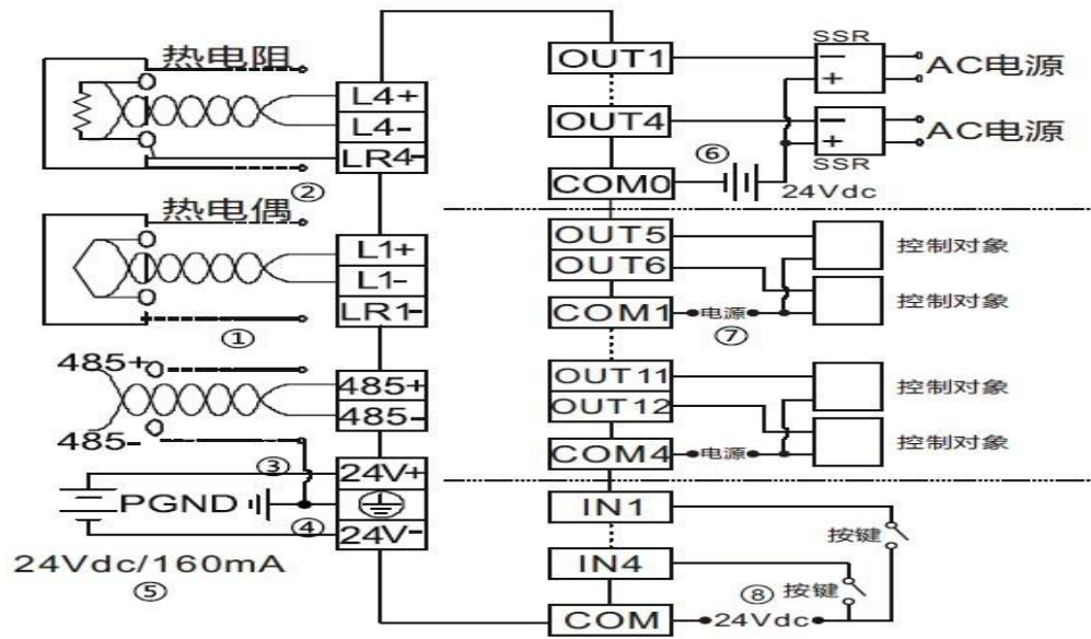
图2-4 MTC-04-NTR输入用户端子布线示意图
