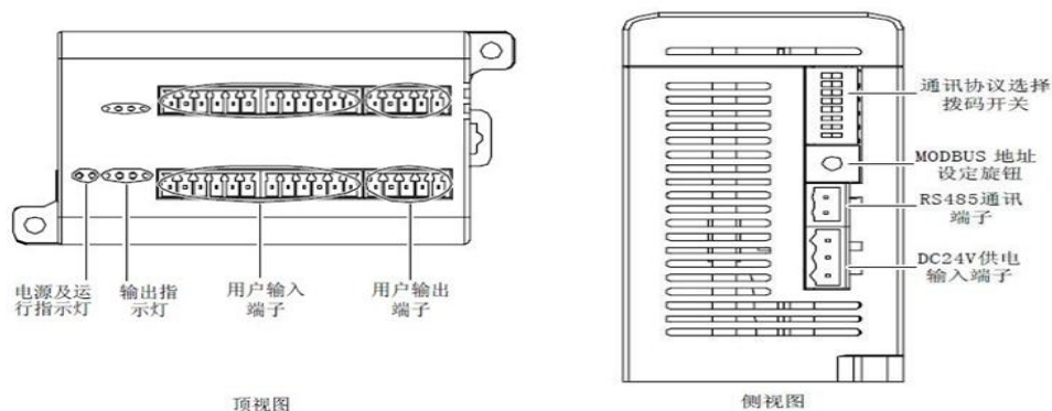
图1-1 MTC-04-NTR外形结构图
