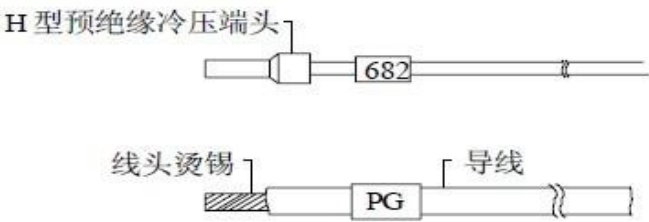
图2-5 MTC 连接电缆制备方式推荐 将加工好的电缆头用螺丝固定在MTC的接线端子上，注意螺钉位置正确，螺钉的旋紧力矩在0.5~0.8Nm，保证可靠连接，又不致损坏螺丝。
