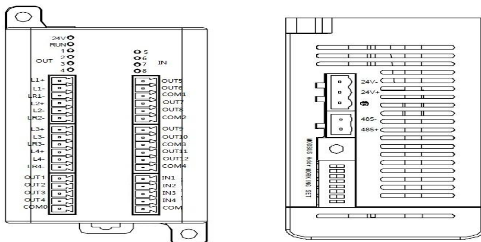
图1-3MTC-04-NTR用户端子图
