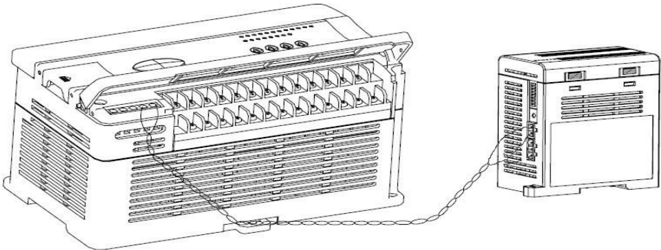
图2-6 连接通讯线 2. 以RS485 方式接入Modbus 主站系统。通过通讯线缆连接MTC的RS485+和RS485-端子到Modbus 主站系统。 注意：1. MTC通讯线的连接方法在不同的系统配置情况下稍有不同。本文以连接MTC与MEGMEET的PLC主模块为例进行说明。其它情况下的通讯线连接请参照进行。 2. 将MTC接入系统后，通过主模块Modbus 或Mdbus 通讯均可读写BFM 区单元。
