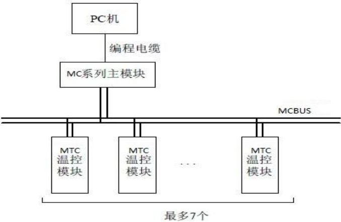
图3-2 连接示意图
