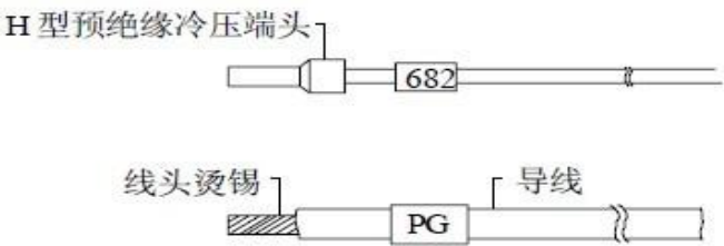
图2-5 MTC 连接电缆制备方式推荐
