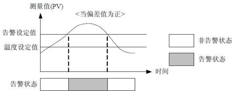
图5-8 上限偏差告警示意图（偏差值为正）
