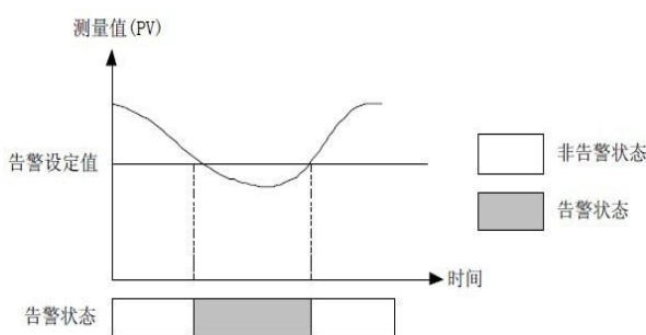
图5-7 下限输入值告警示意图
