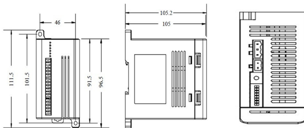
图1-2MTC-04-NT安装尺寸图（单位：mm）
