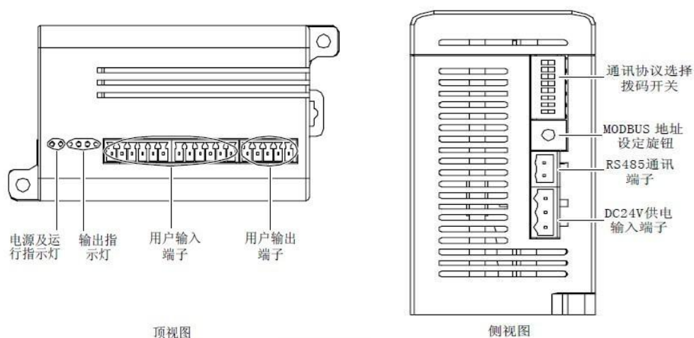
图1-1 MTC-04-NT外形结构图
