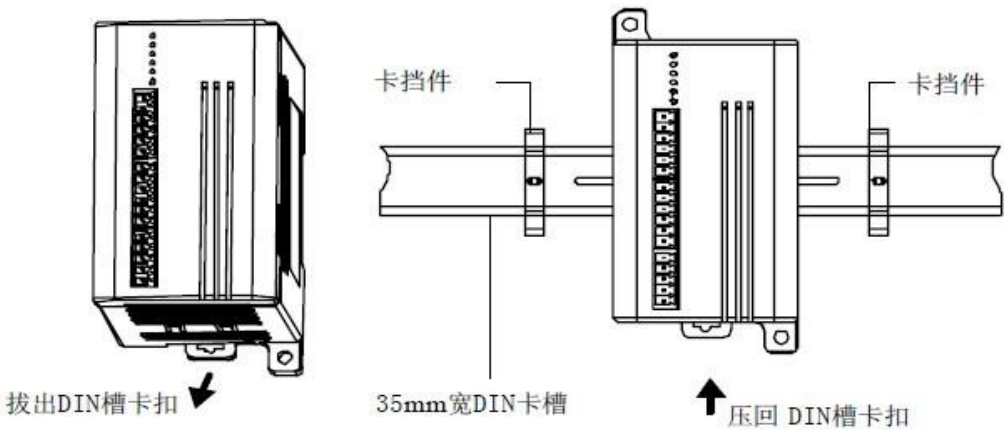
图2-2 采用DIN 槽安装固定
