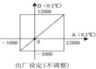
图5-2 不更改各通道的D0、D1 值，对应通道特性（以模式3 示例）
