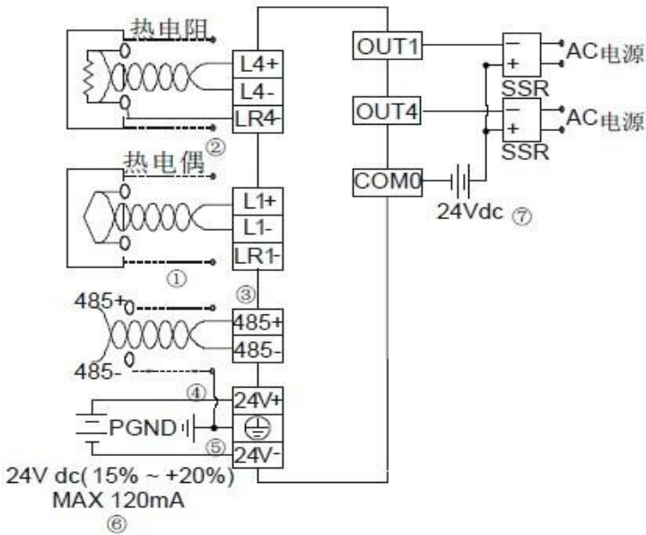
图2-4 MTC-04-NT输入用户端子布线示意图
