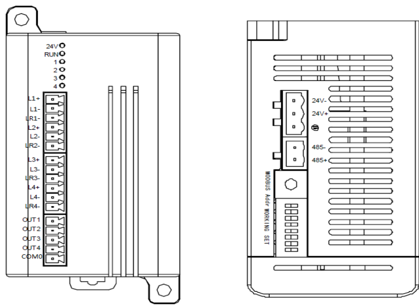
MTC-04-NT用户端子如图1-3所示
