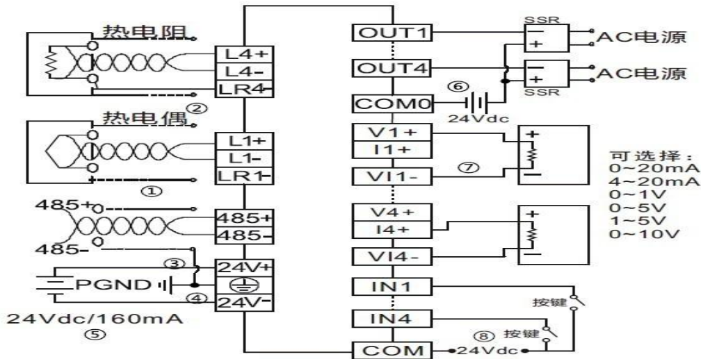
图2-4 MTC-04-NVT输入用户端子布线示意图
