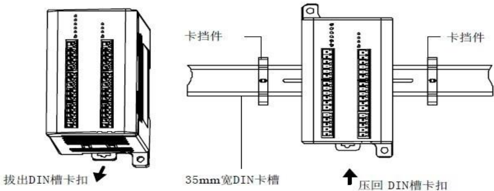
图2-2 采用DIN 槽安装固定
