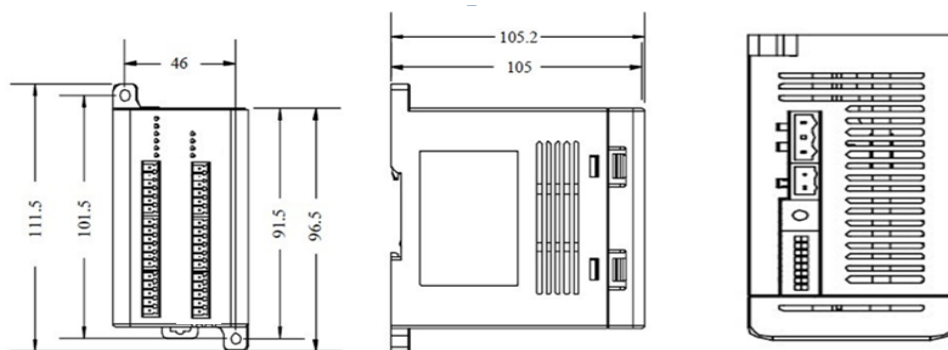
图1-2MTC-04-NVT安装尺寸图（单位：mm）
