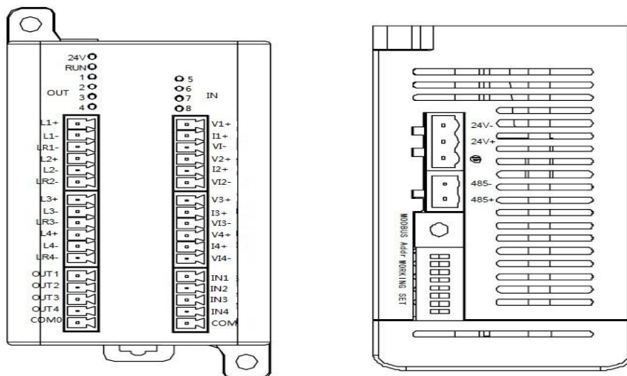
图1-3MTC-04-NVT用户端子图
