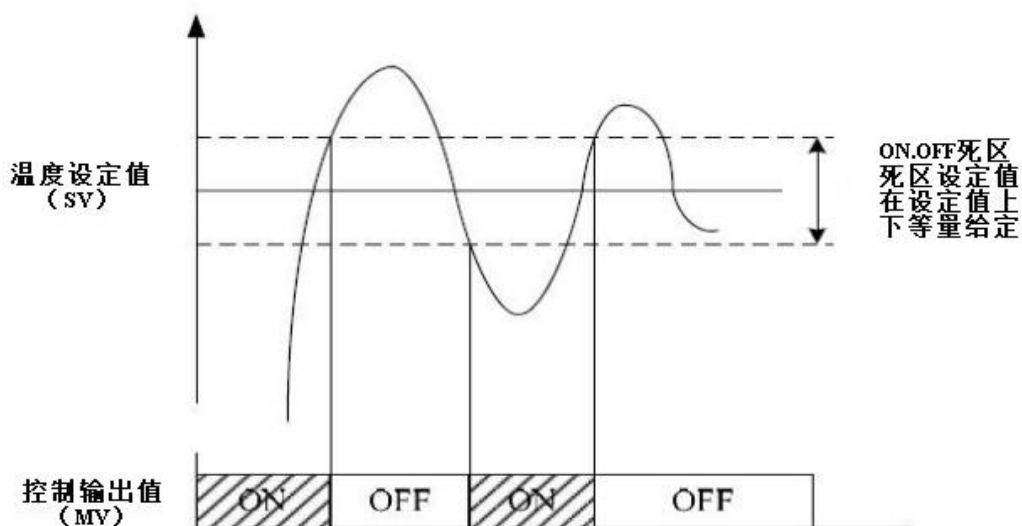
图 4-3 ON/OFF 控制
