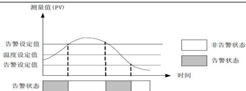
图 4-21 范围告警示意图
