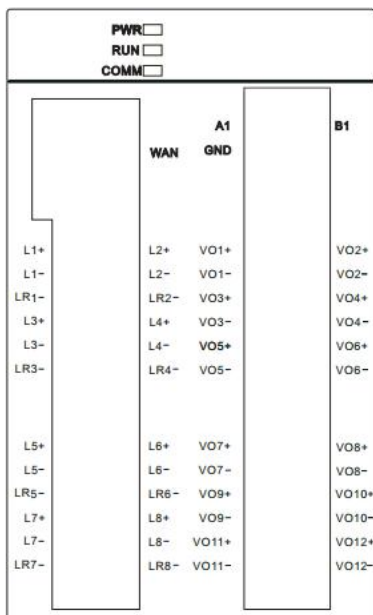
图 1-5 MTCW-08-NV 用户端子图
