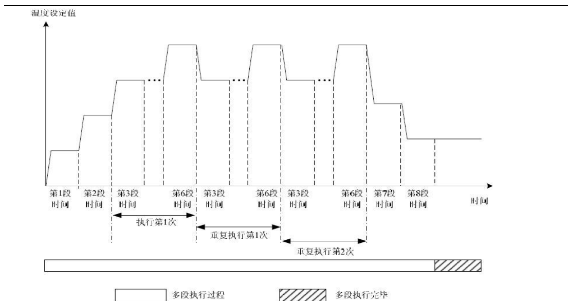
图 4-10 多段设定值执行示意图
