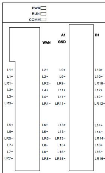
图 1-7 MTCW-16-NN 用户端子图
