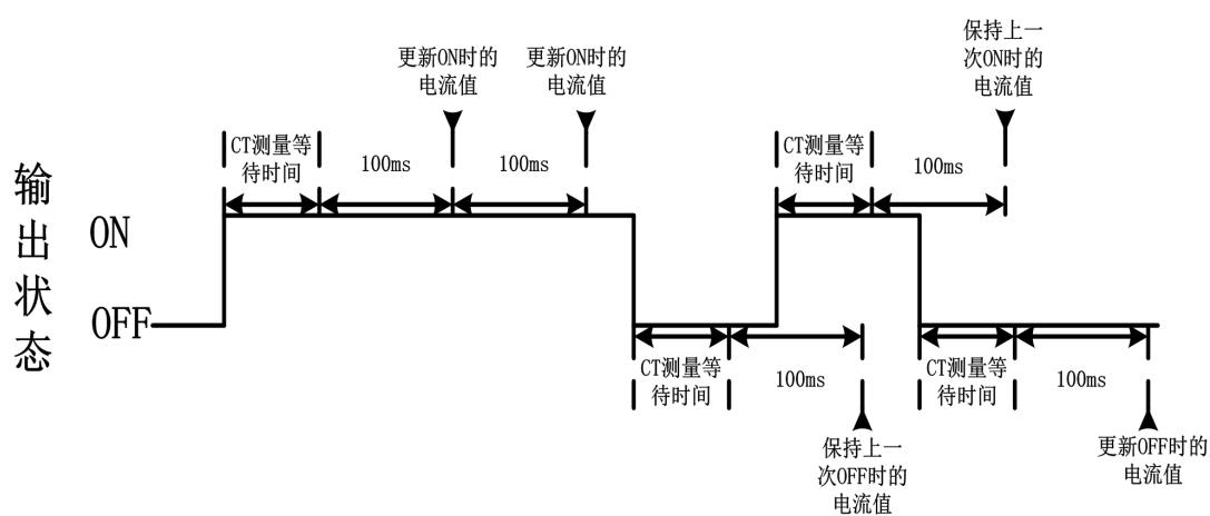
图 4-29 CT 更新时间
