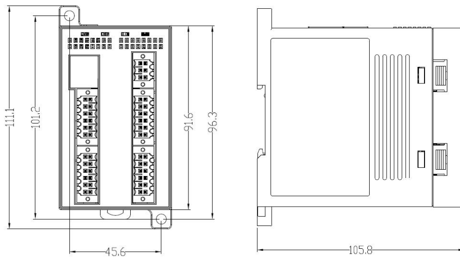
图 1-2 MTCW 安装尺寸图 ( 单位 : mm )
