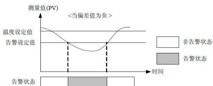
图 4-19 偏差下限告警示意图 ( 偏差值为负 )
