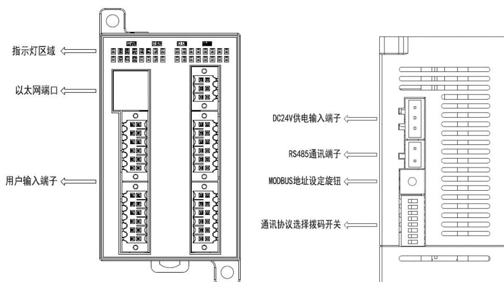
图 1-1 MTCW 外形结构图
